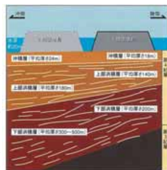
空港島建設海域の地盤の様子
